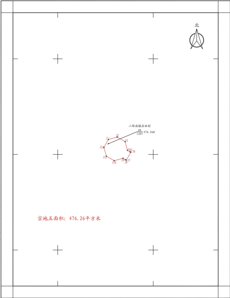
南阳方城风电场一期工程改造升级项目勘测定界图宗地五
