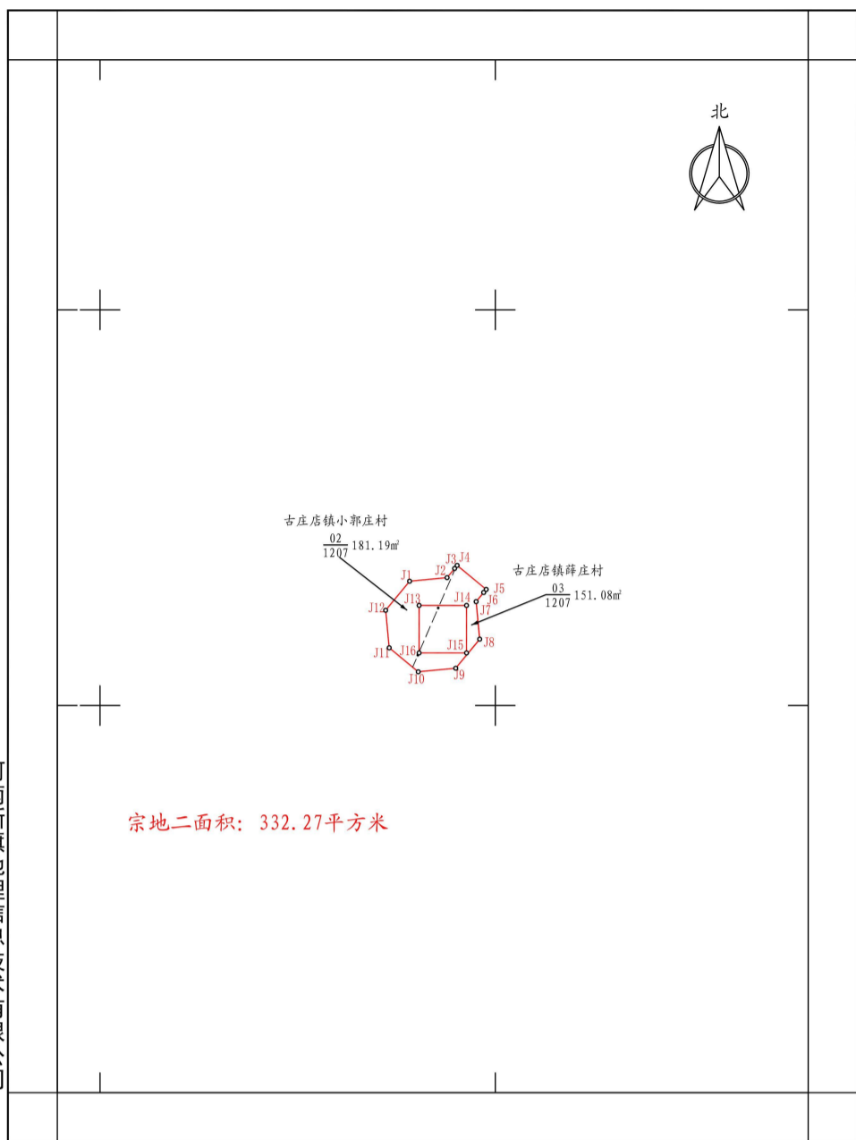
南阳方城风电场一期工程改造升级项目勘测定界图宗地二
