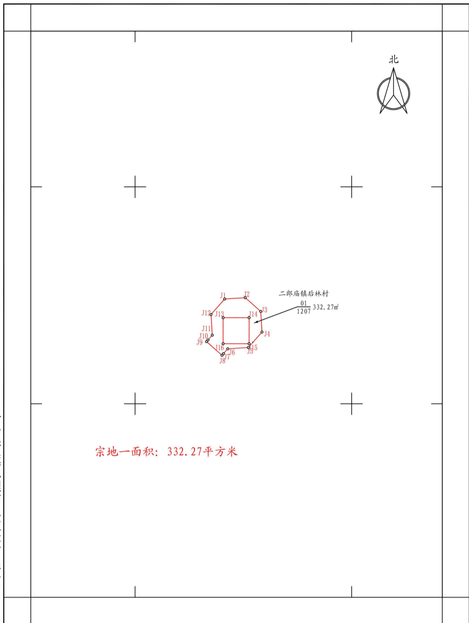
南阳方城风电场一期工程改造升级项目勘测定界图宗地一
