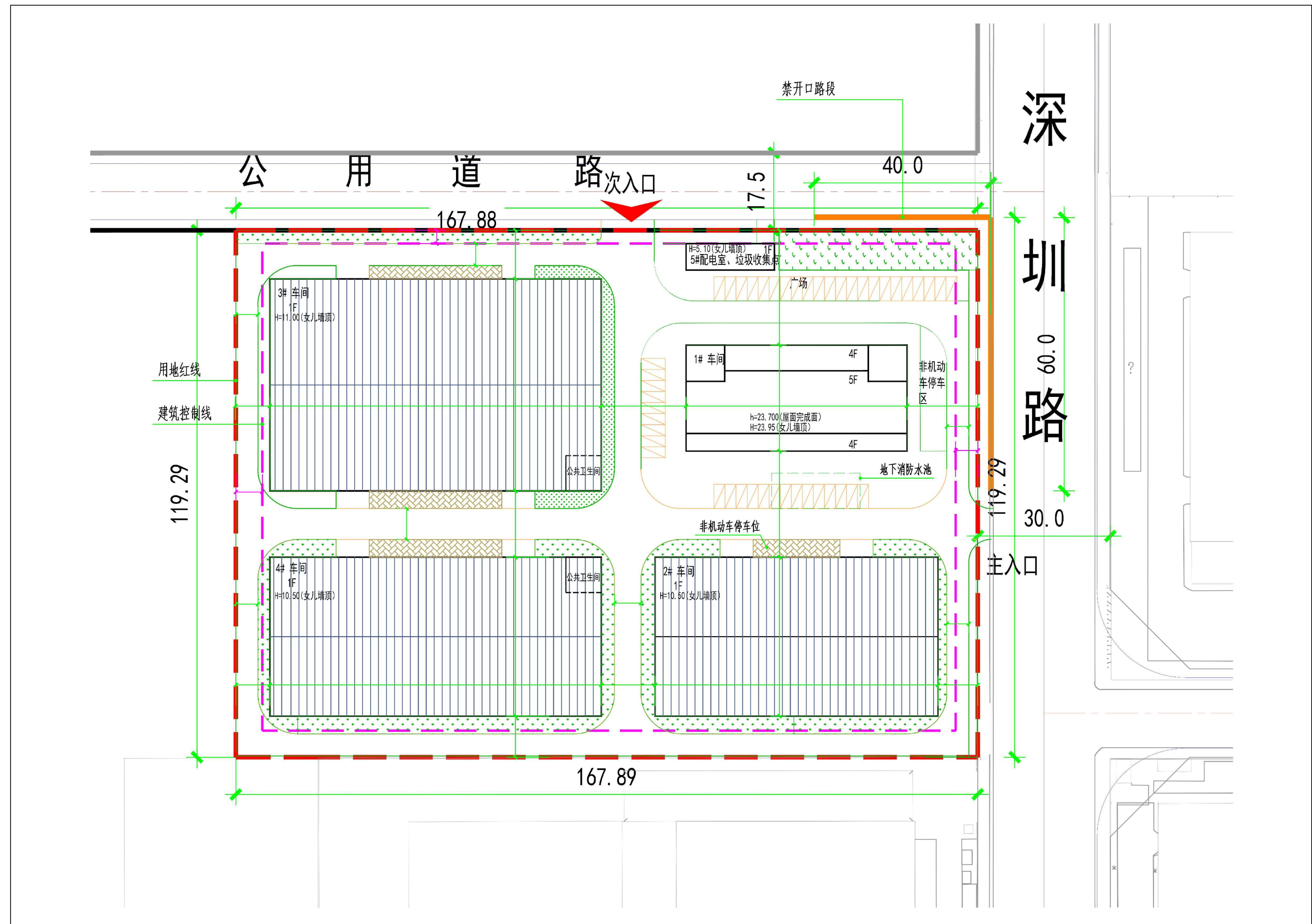
总平面图
