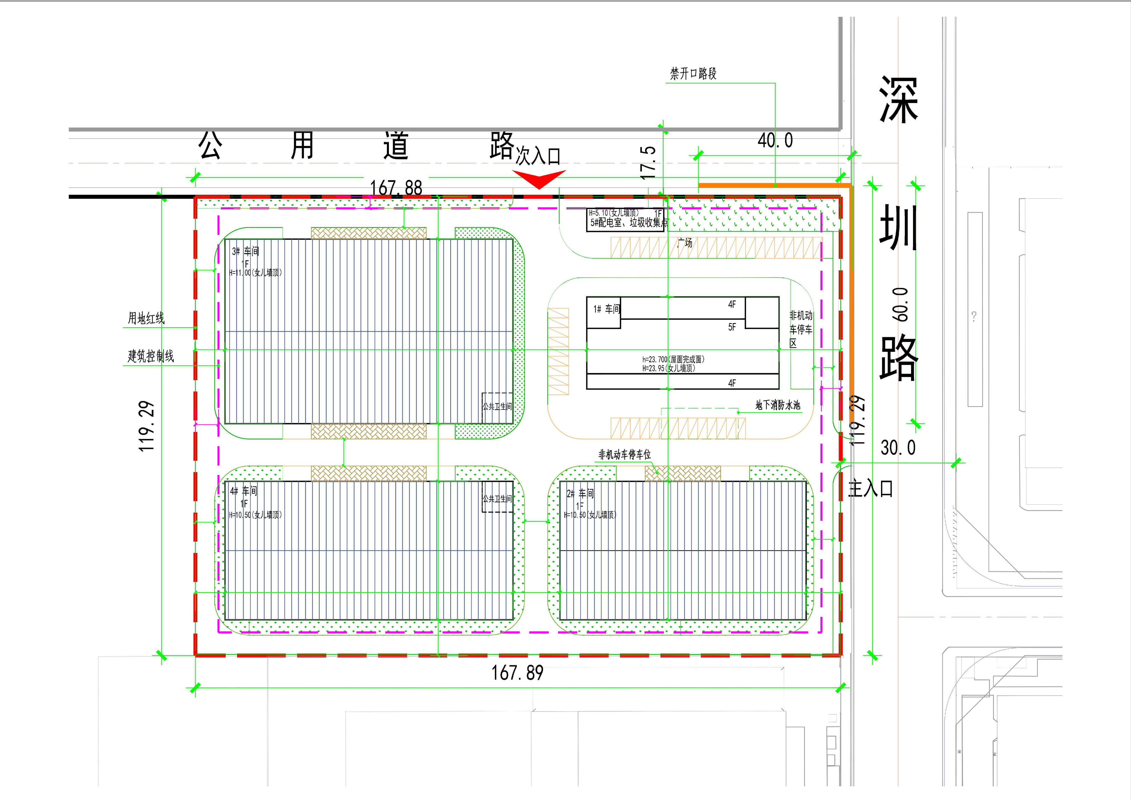
规划平面图
