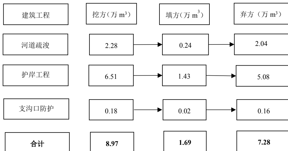
图 3 土方平衡流向框图
