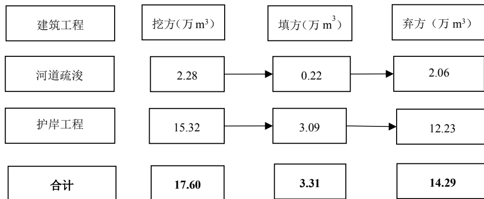
图 3 土方平衡流向框图
