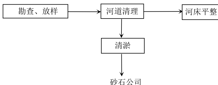
图 1 施工期河道清淤疏浚工程工艺流程及产污环节图
